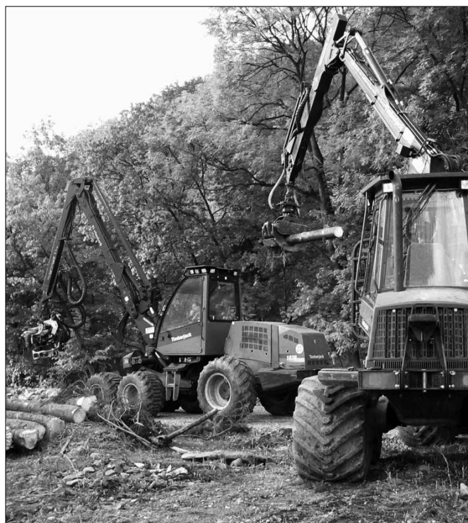
Moderne Forstmaschinen, wie Harvester und Forwarder, die zur hochmechanisierten Holzernte eingesetzt werden, stellt der Staatsbetrieb Sachsenforst zum Landeserntedankfest in Frankenberg vor.
